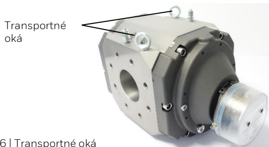
Obr. 6 | Transportné oká
