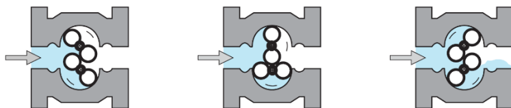
Obr. 1b | Funkčný princíp rotačného piestového plynomeru
