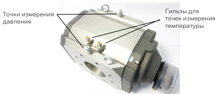
Рис. 5 | Точки измерения температуры и давления
