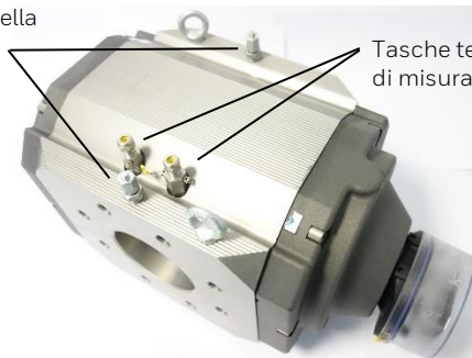
Fig. 5 | Prese di misura della temperatura e della pressione
