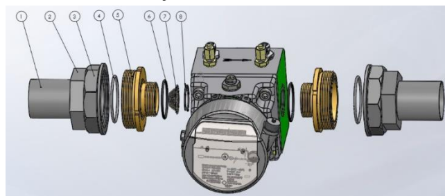
Fig. 8 | Raccordi tipo RABO-CT
