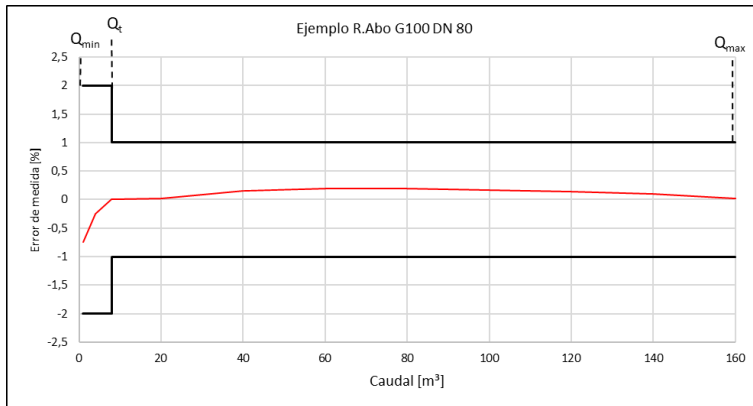
Fig. 13 | Límites de error
