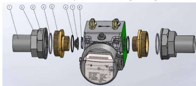
Afb. 8 | Anschlussteile Typ RABO-CT
