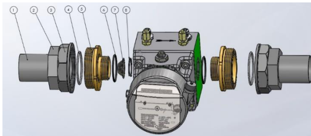
Fig. 8 | Éléments de raccordement type RABO-CT
