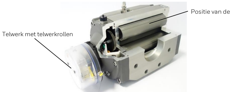
Afb. 9 | RABO-doorsnede
