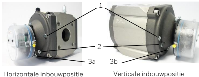
Afb. 12 | Inbouw-, onderhouds- en controleposities
