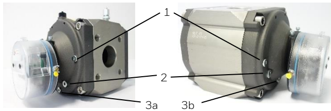
Position de montage horizontale
