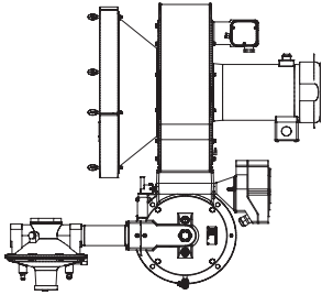
Tubería derecha
