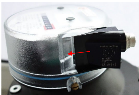
Afb. 1 | Installatie IN-Sxx
