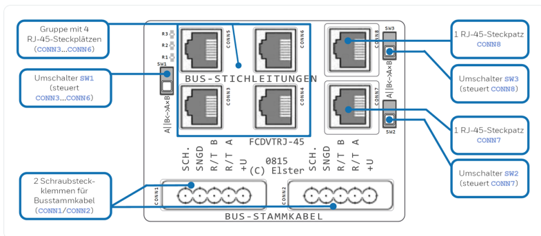
Abb. 2-1: DSfG-Verteiler RJ-45 FCDVTRJ-45
