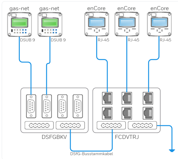
Abb. 2-2: DSFGBK und FCDVTRJ-45 miteinander koppeln
