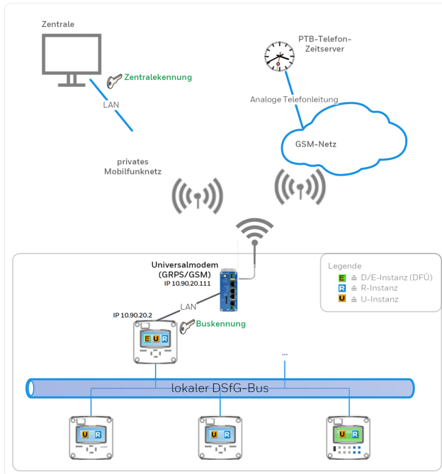
Abb. 3-2: Klasse B über das Universalmodem – Beispiel DFÜ-Instanz mit einer Zentrale (GPRS) und Zeitabgleich über den PTB-Telefon-Zeitserver (GSM)
