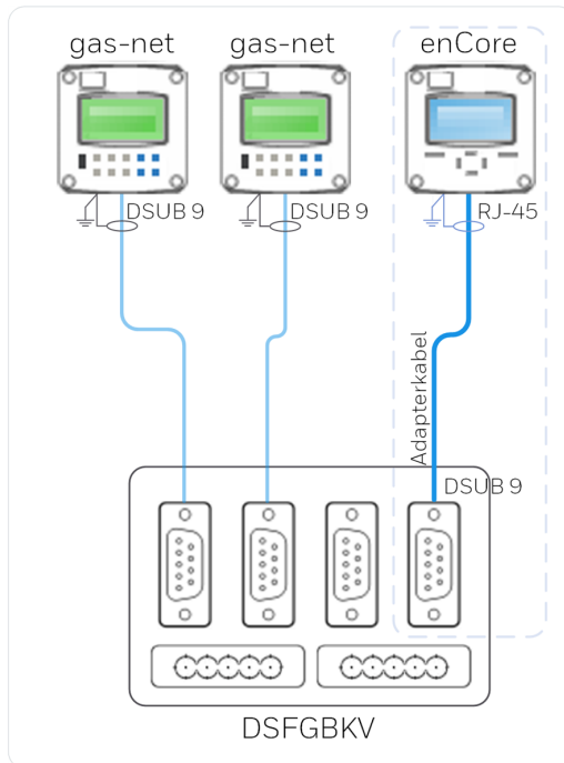
Abb. 2-4: enCore-Gerät direkt mit DSfGBKV verbinden – Beispiel
