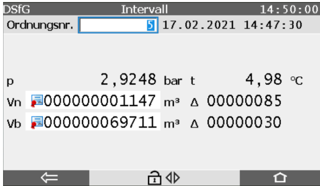
Abb. 4-4: Archivgruppe Intervall – Beispiel
