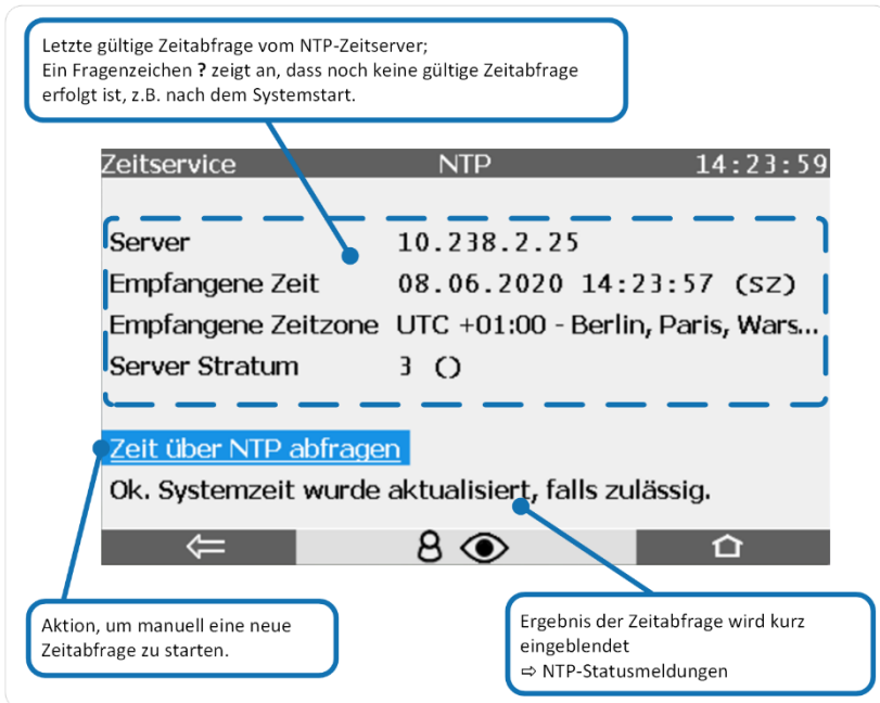
Abb. 5-9: Anzeige NTP – Beispiel
