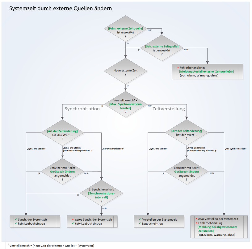
Abb. 5-3: Funktionsweise und Parametrierung der externen Zeitquellen in der Übersicht
