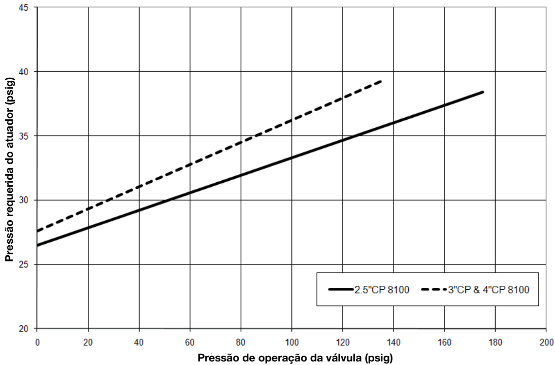
Pressão requerida para o atuador Série 8100: 2,5" CP, 3" CP, 4" CP
