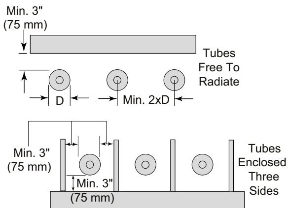
Fig. 5. SER Burner Sizing Example
