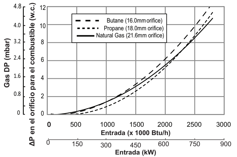
\Delta P en el orificio para el combustible frente a entr
