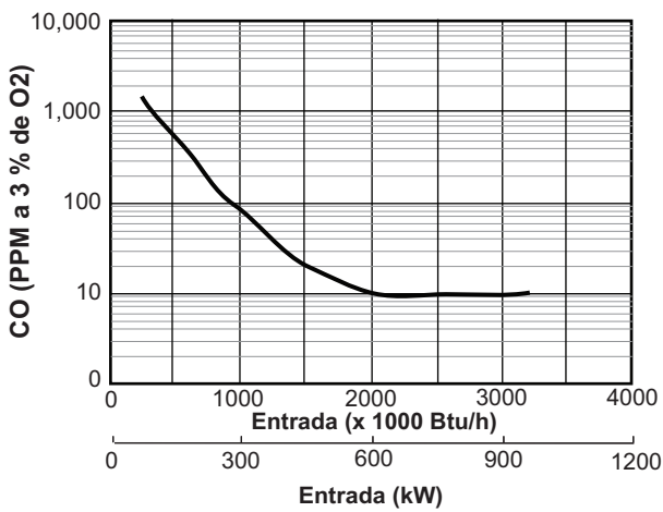
Curva de CO característica
