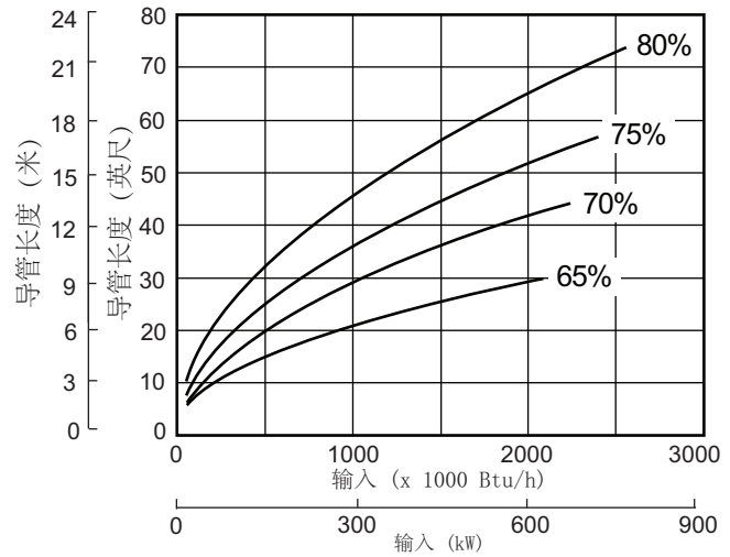
热传递与导管长度 (以百分比表示各种效率)
