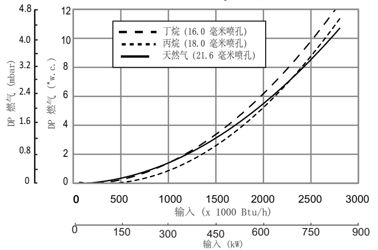
燃料喷嘴 \Delta p 与输入
