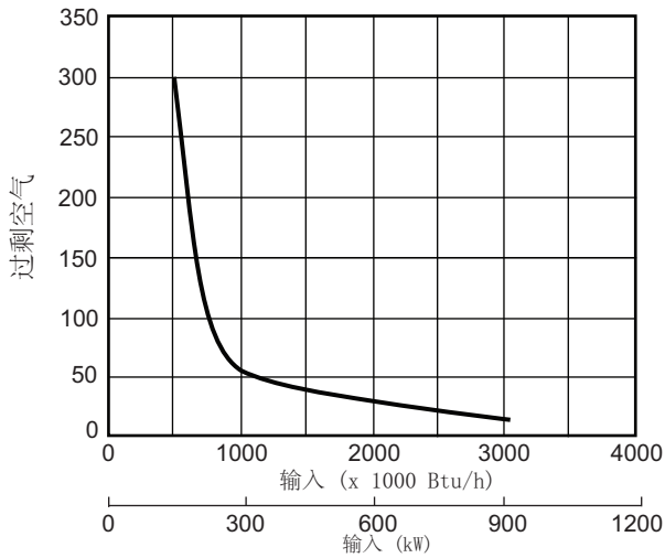
控制和运转曲线
