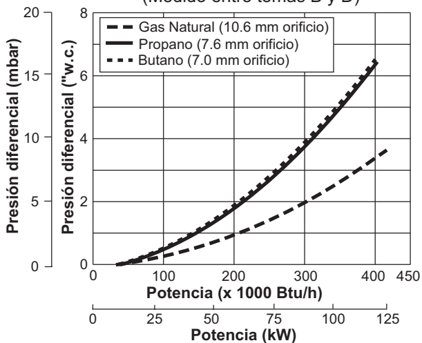
\Delta P Diafragma de gas vs. Potencia - 6" w.c. Ventilador (Medido entre tomas B y D)
