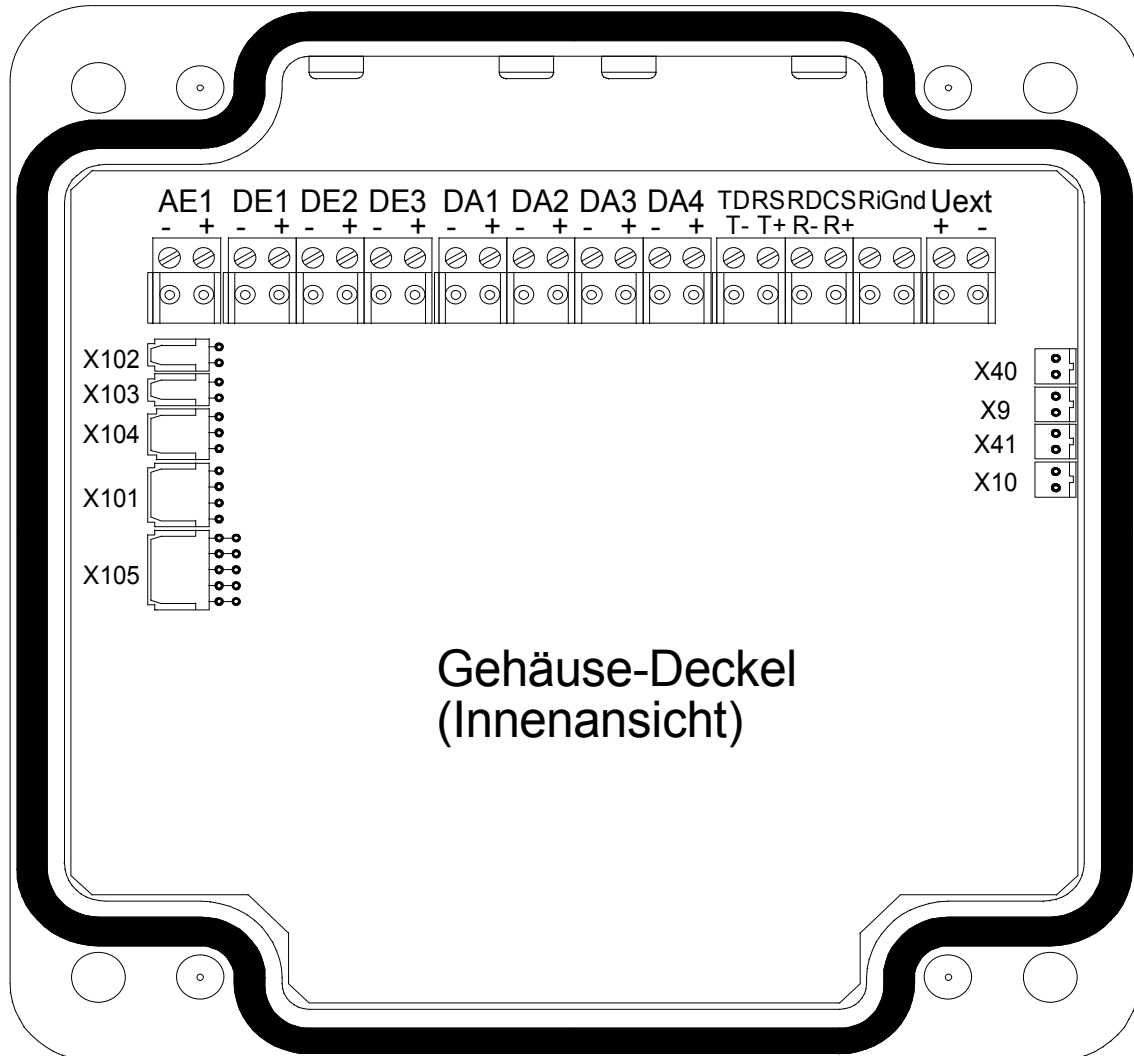
Abbildung 4: Anschlussplan
