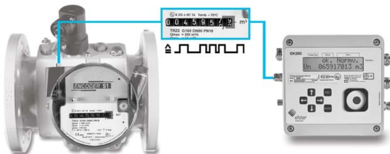
Représentation schématique de la transmission de l'index original au convertisseur de volume à pile EK260 par l'interface NAMUR
